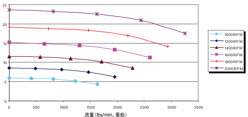
Metallics D-13XL搬送ポンプの性能(亜鉛の場合)
